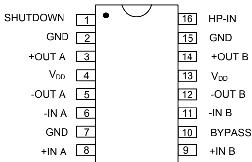
DIP-16/SOP-16
