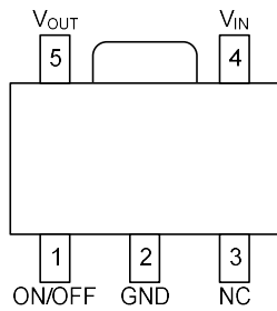
SOT-89-5
