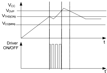
Fig.4 OVP case
