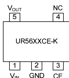
SOT-23-5 / SOT-25
