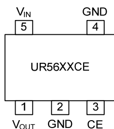
SOT-23-5
